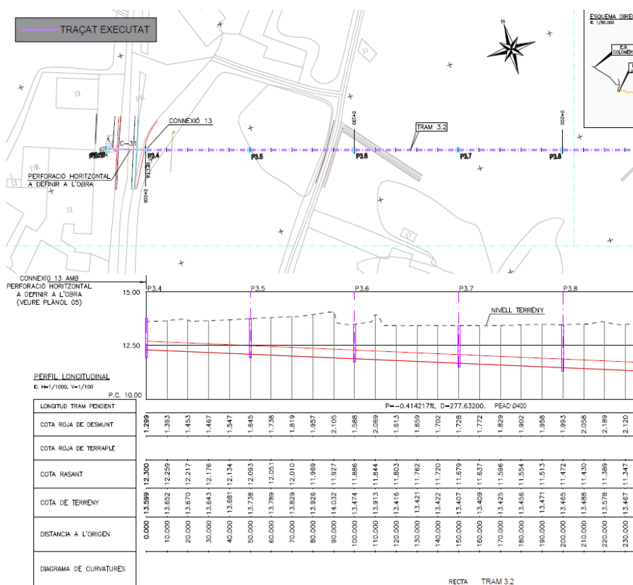
Figura 3. Detall del plànol planta i perfil longitudinal del col·lector "Tram 3.2" del projecte d'obra executada
