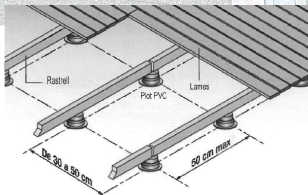
DETALL ORIENTATIU DE L'ESTRUCTURA SOBRE PLOTS
