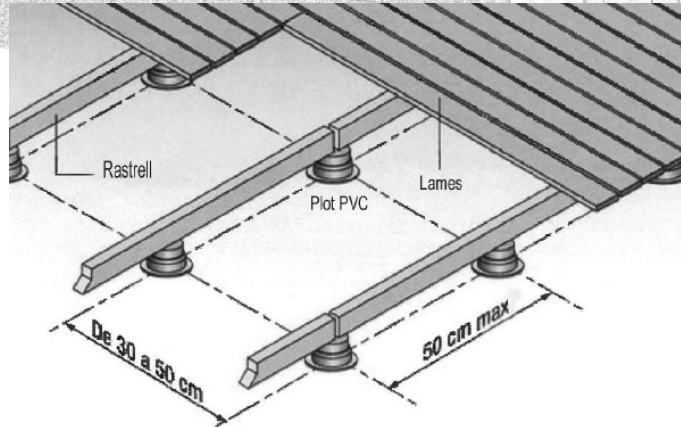
DETALL ORIENTATIU DE L'ESTRUCTURA SOBRE PLOTS
