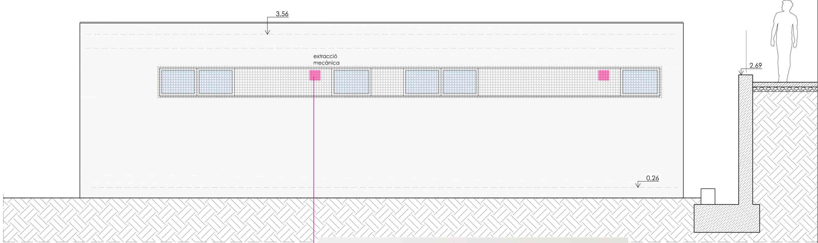
FAÇANA DAVANTERA/CAMP DE FUTBOL e.: 1/50
