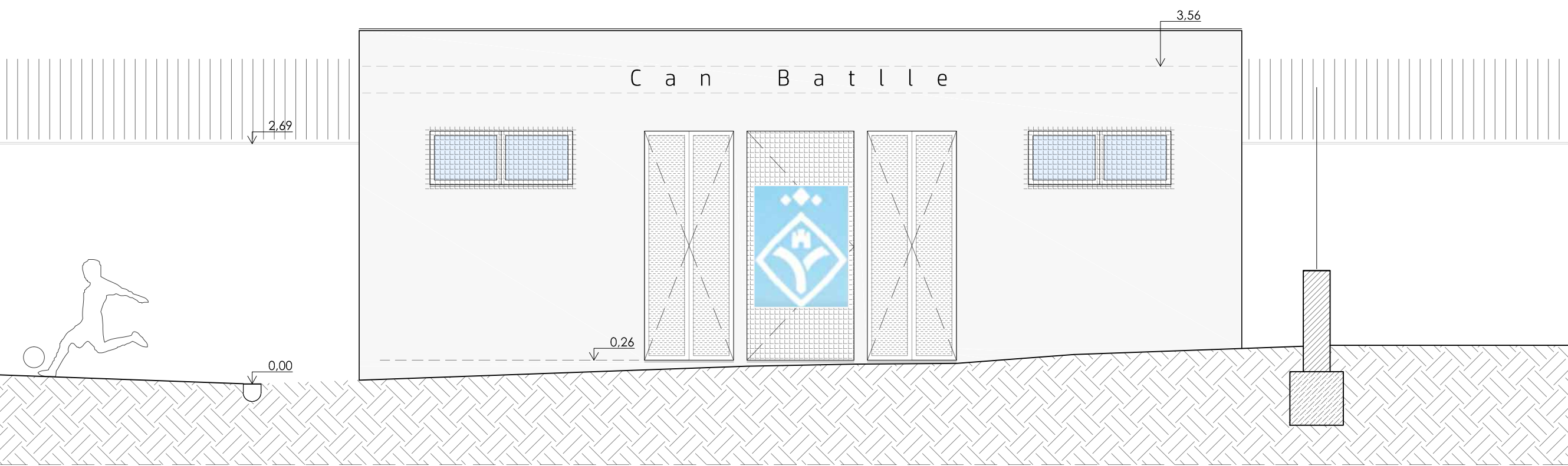
FAÇANA LATERAL DRETA e.: 1/50
