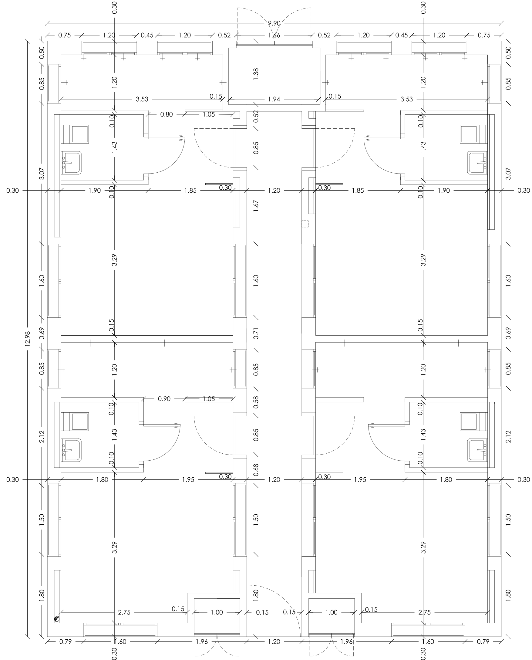
PLANTA COTES e.: 1/50
