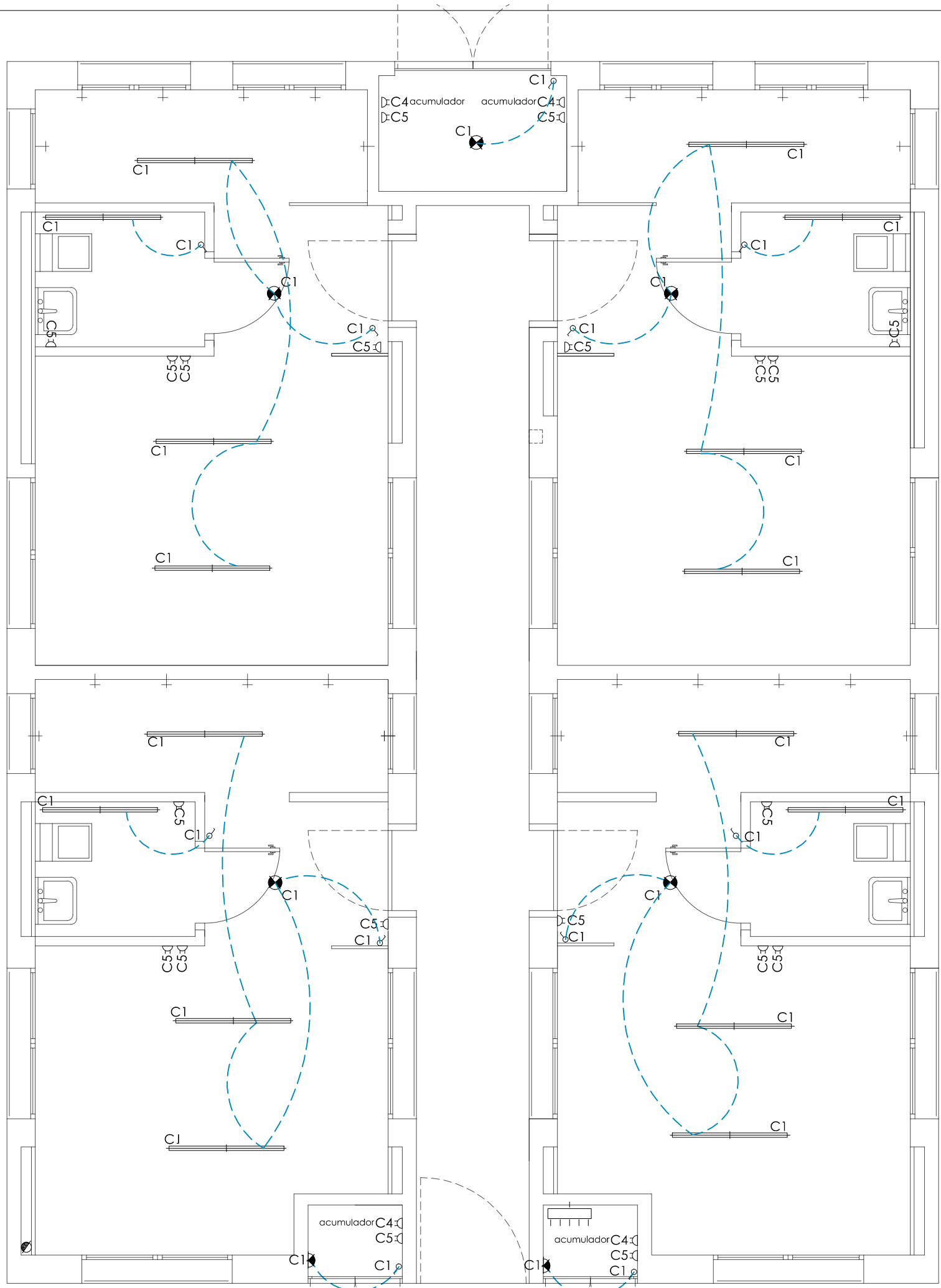
ESQUEMA INST. ELÈCTRICA e.: 1/50
