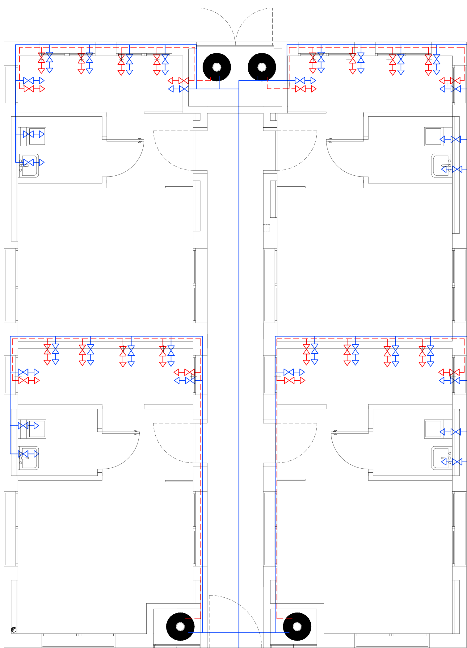
ESQUEMA INST. LLAUNERIA e.: 1/50
