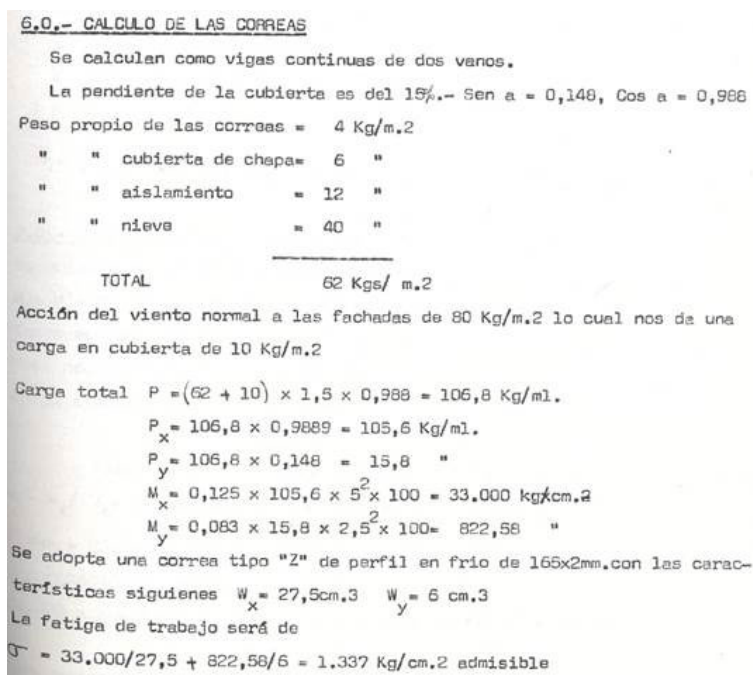
Fig. 6.1. Càlcul original de càrregues estructurals
