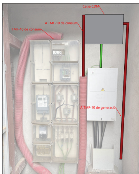
Fig. 7.4. Disposició CDM dins la TMF-10.
