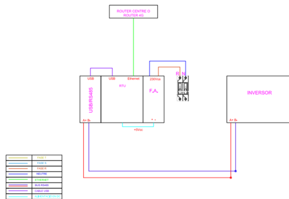
Fig. 7.2. Diagrama unifilar del sistema de monitoratge.
