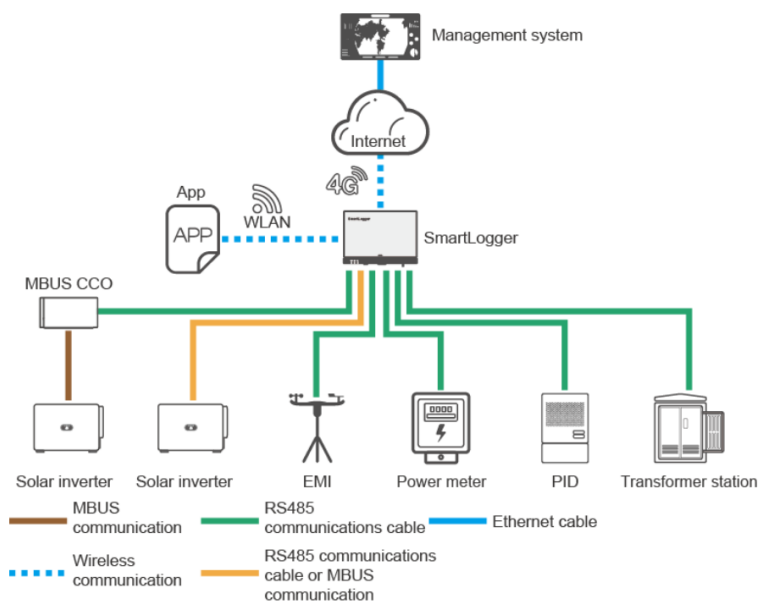
Fig. 7.1. Connexió i funcionament del sistema de monitoratge.
